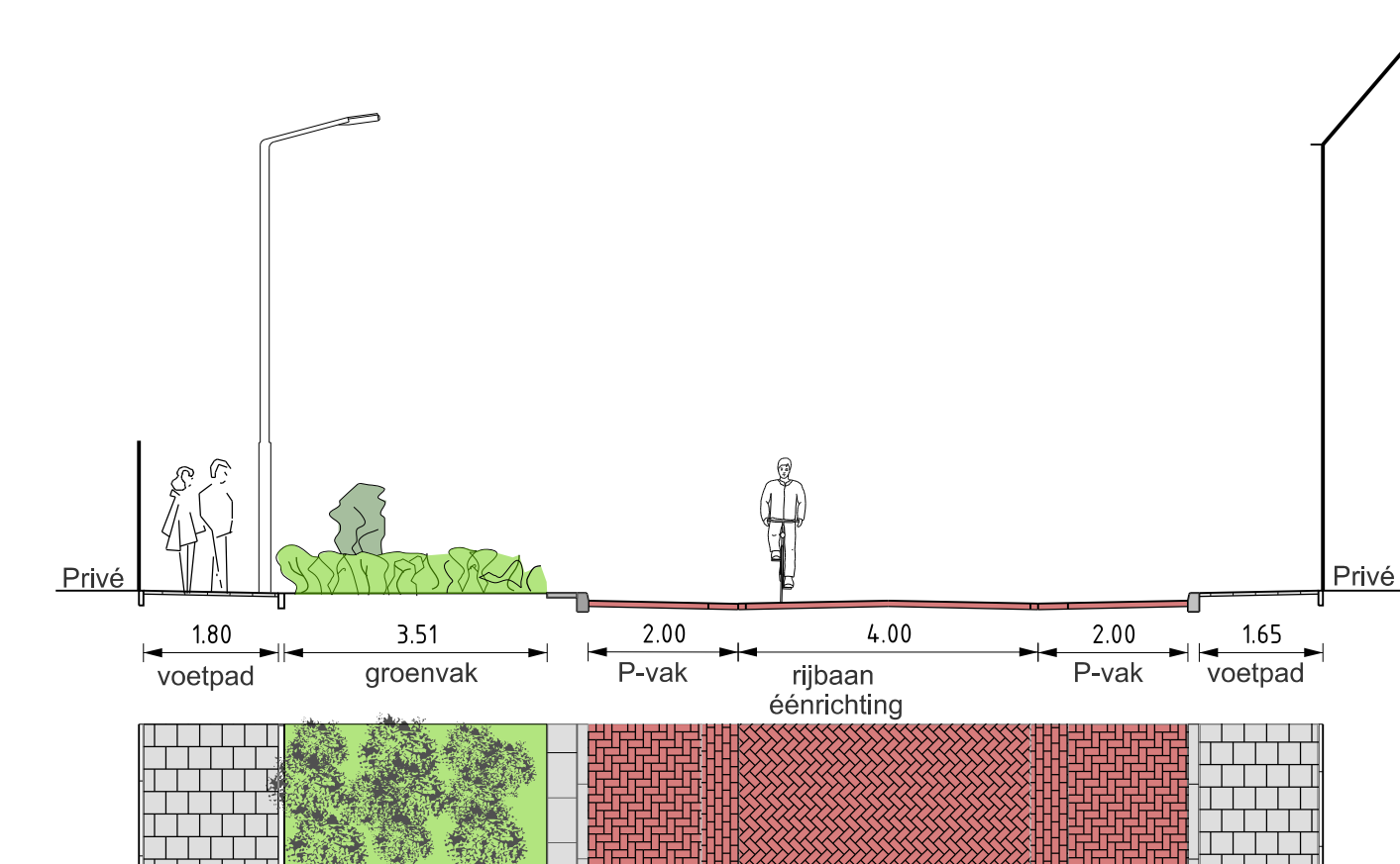
DOORSNEDE C-C' 1 : 100
