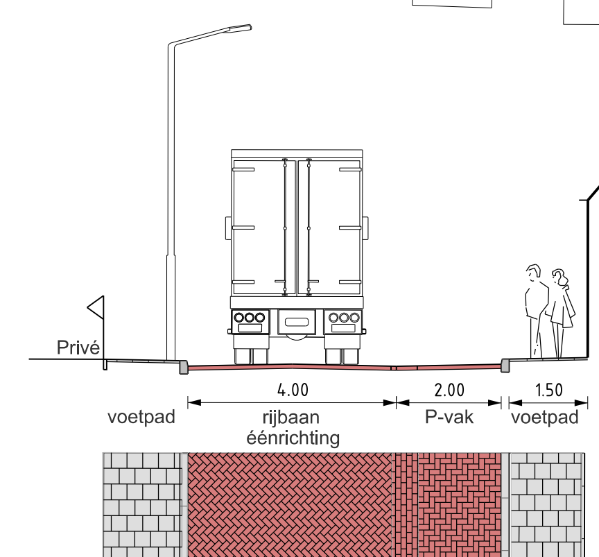
DOORSNEDE A-A' 1 : 100
